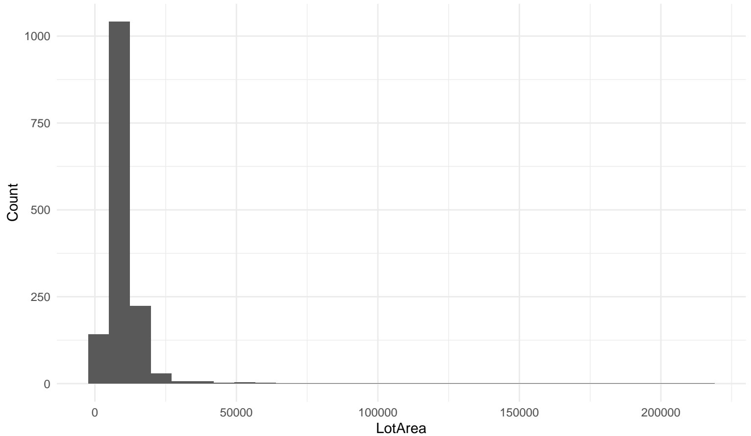
Histogram: LotArea
