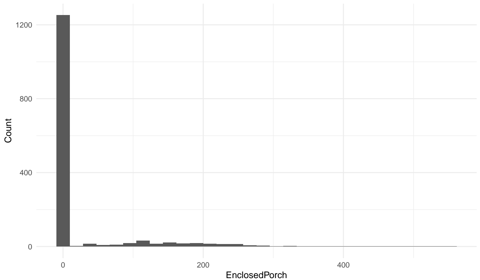
Histogram: EnclosedPorch
