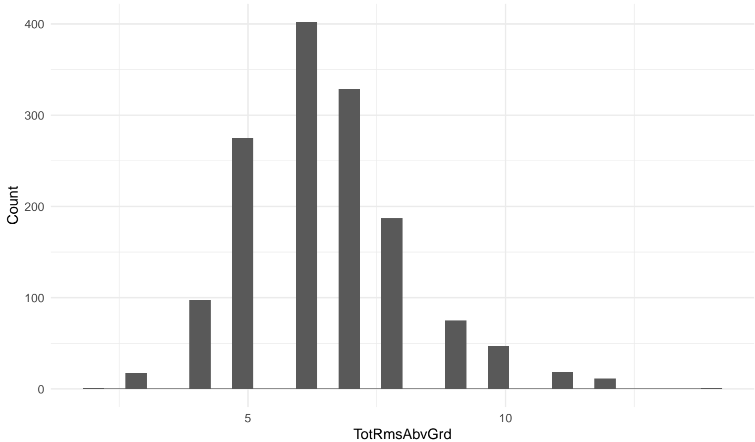
Histogram: TotRmsAbvGrd
