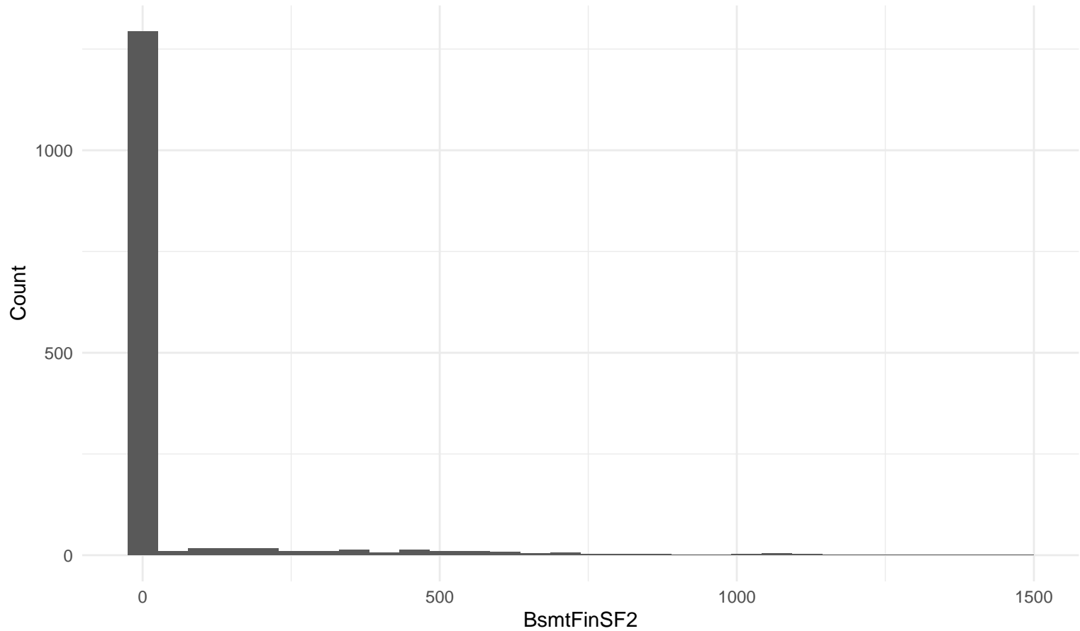
Histogram: BsmtFinSF2
