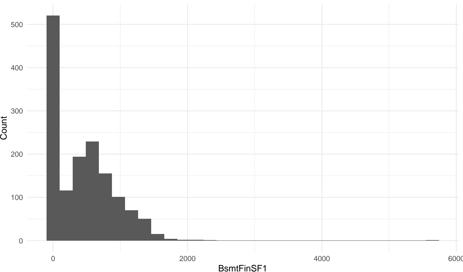
Histogram: BsmtFinSF1
