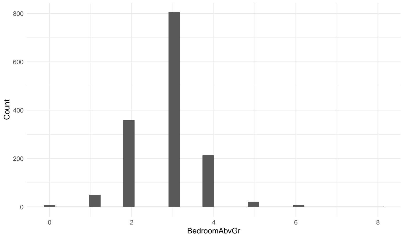
Histogram: BedroomAbvGr
