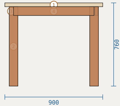
VEDERE LATERALĂ
