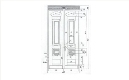
Bestandsplan / Referenz
