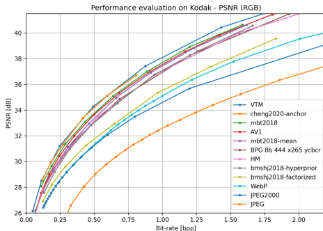
Figura 3: PSNR (RGB) sobre Kodak. Fuente: CompressAI.
