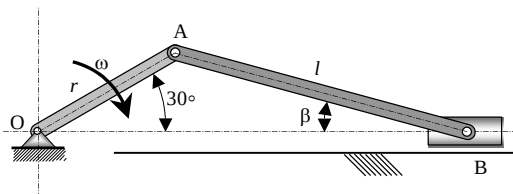
Slika 3.1 Shema motornog mehanizma (OA- pogonska ručica, AB – poluga, B – klizač, itd.)
