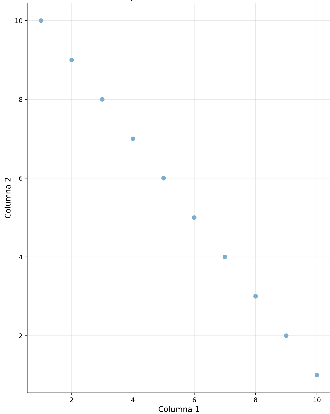
Gráfico de Dispersión: Columna 1 vs Columna 2
