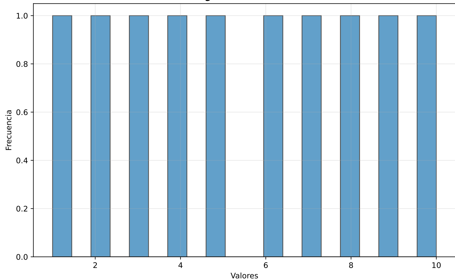
Histograma de Columna 2
