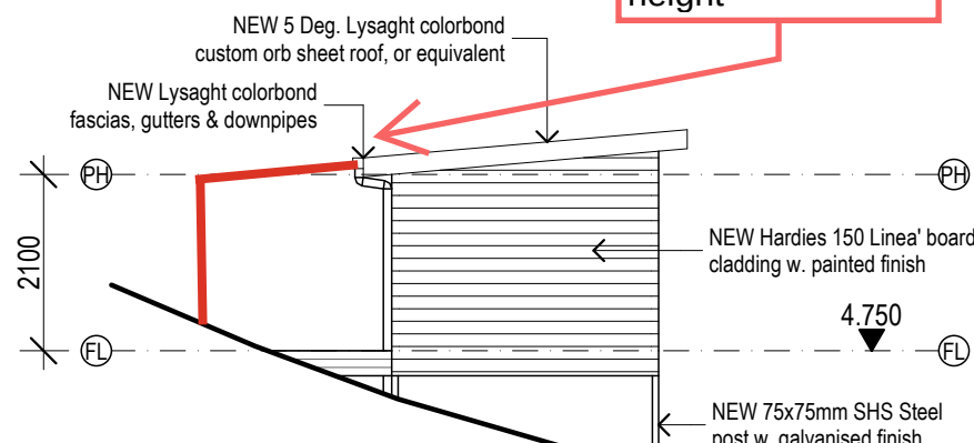
ELEVATION 4 1:100
