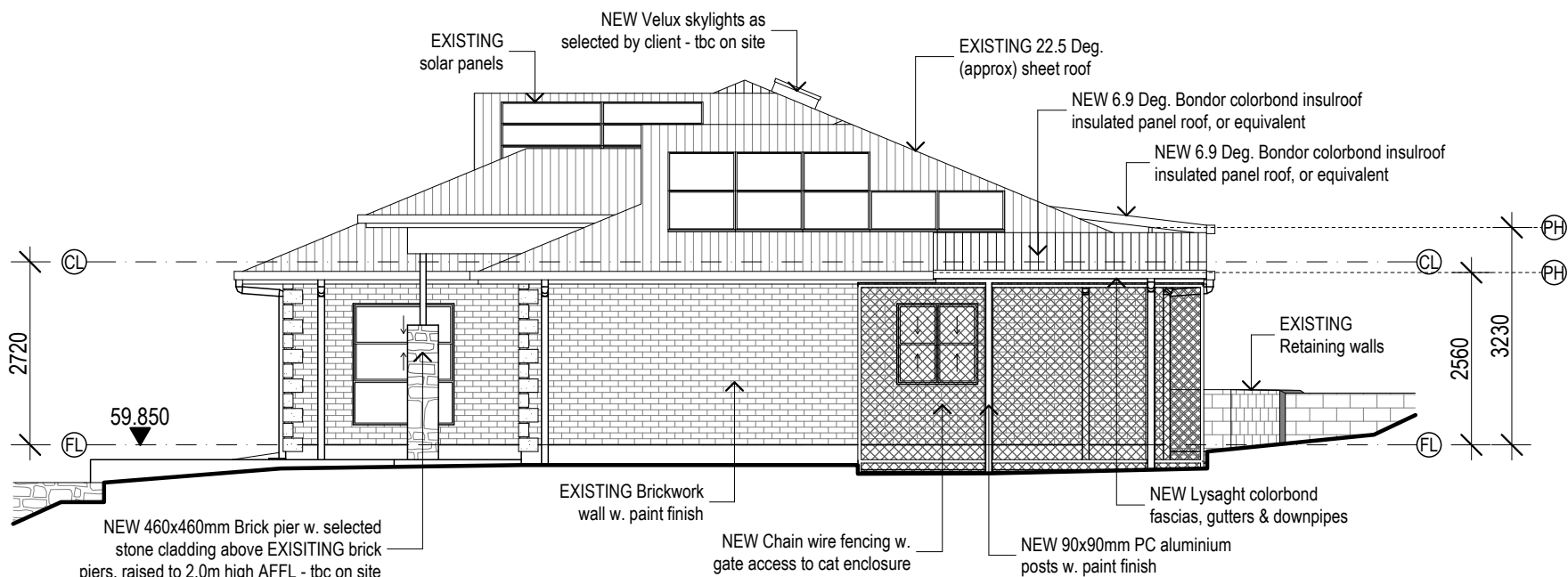
ELEVATION 2 1:100
