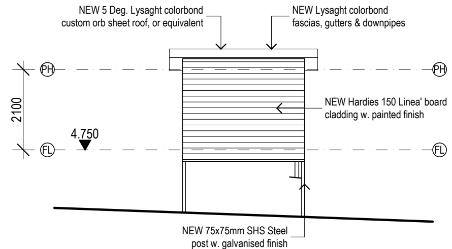
ELEVATION 1 1:100
