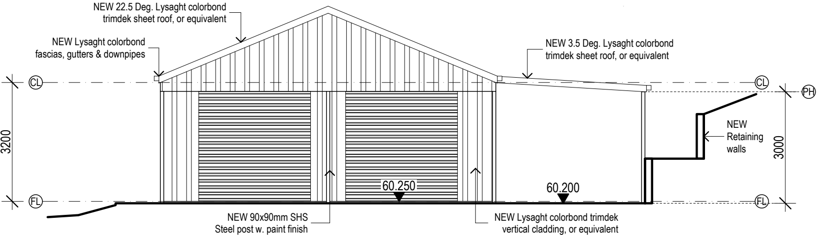
ELEVATION 2 1:100
