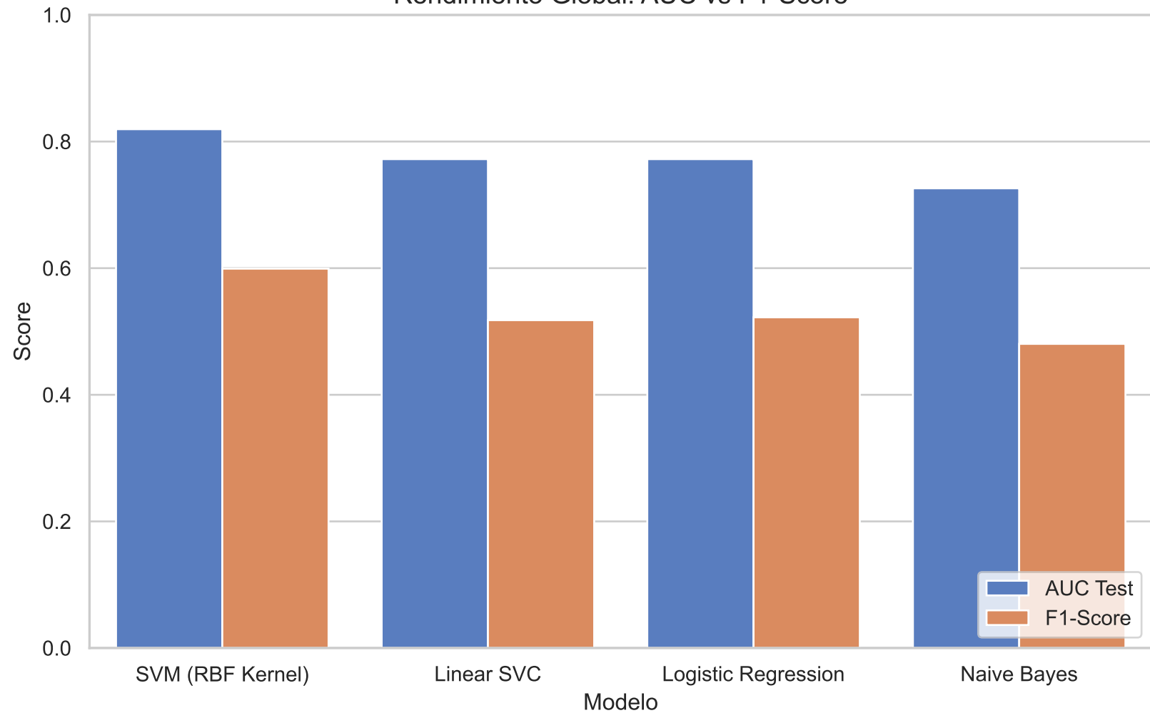
Rendimiento Global: AUC vs F1-Score
