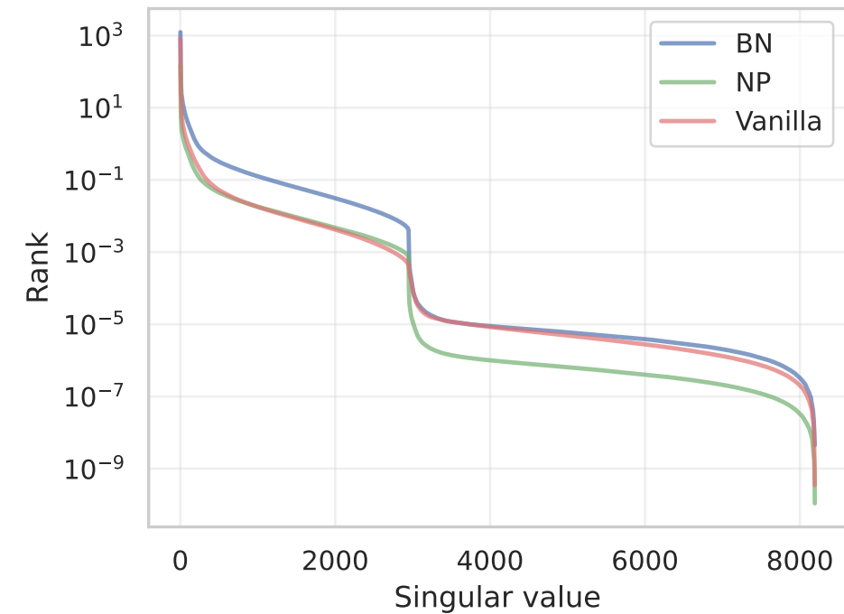
UCI HAR
