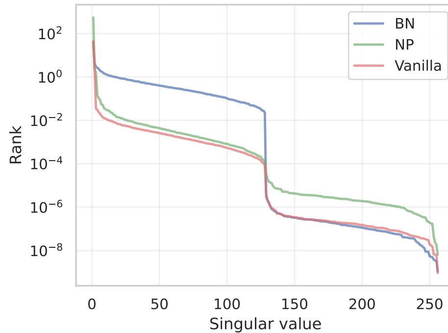
IMDb
