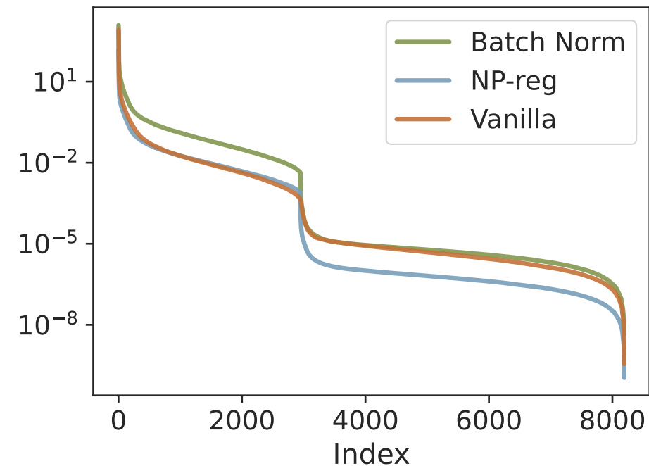
UCI HAR
