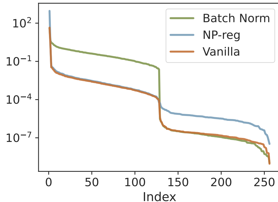
IMDb
