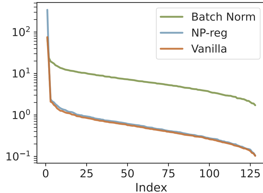
IMDb
