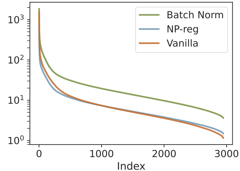
UCI HAR
