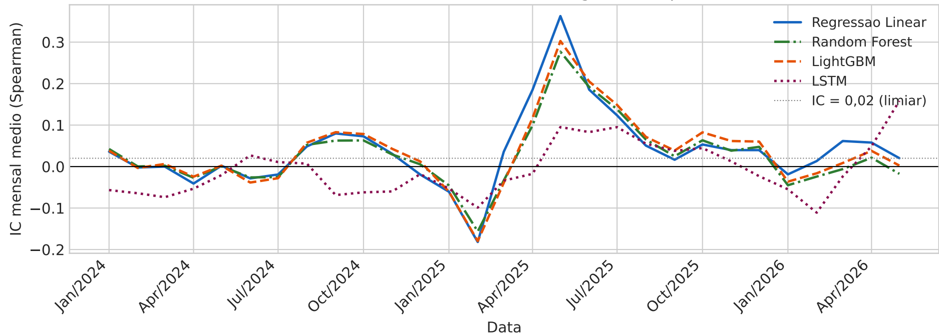
Information Coefficient ao Longo do Tempo
