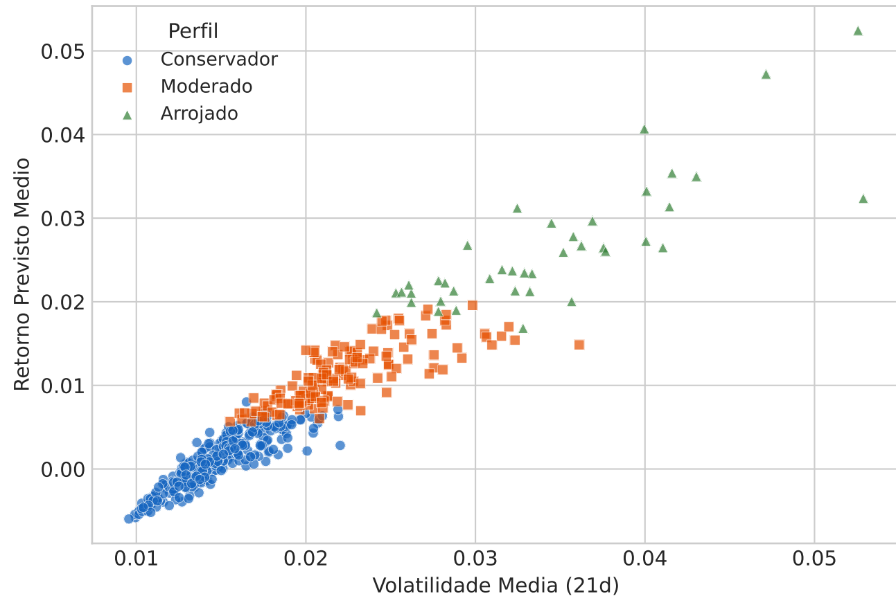
K-Means — Perfis de Investidor (K=3)
