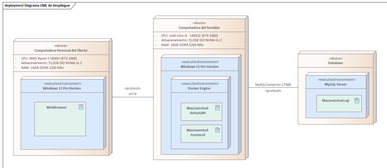
Ilustración 13. Diagrama de despliegue
