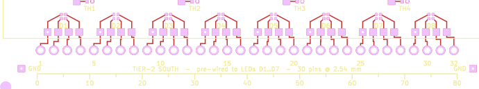
WL-SFCC 0404 RGB LEDs
