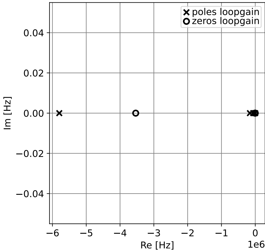
PZplotloopgain
