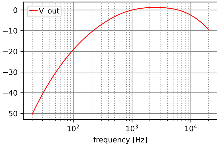
DIN A weighting function
