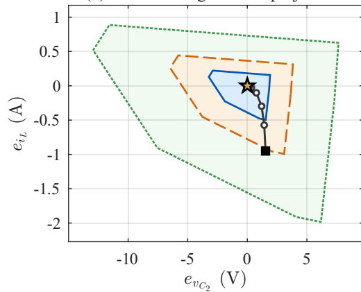
(d) Second voltage-current projection
