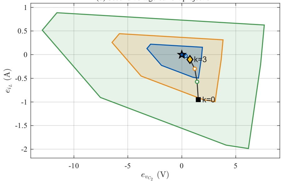
(d) Second voltage-current projection
