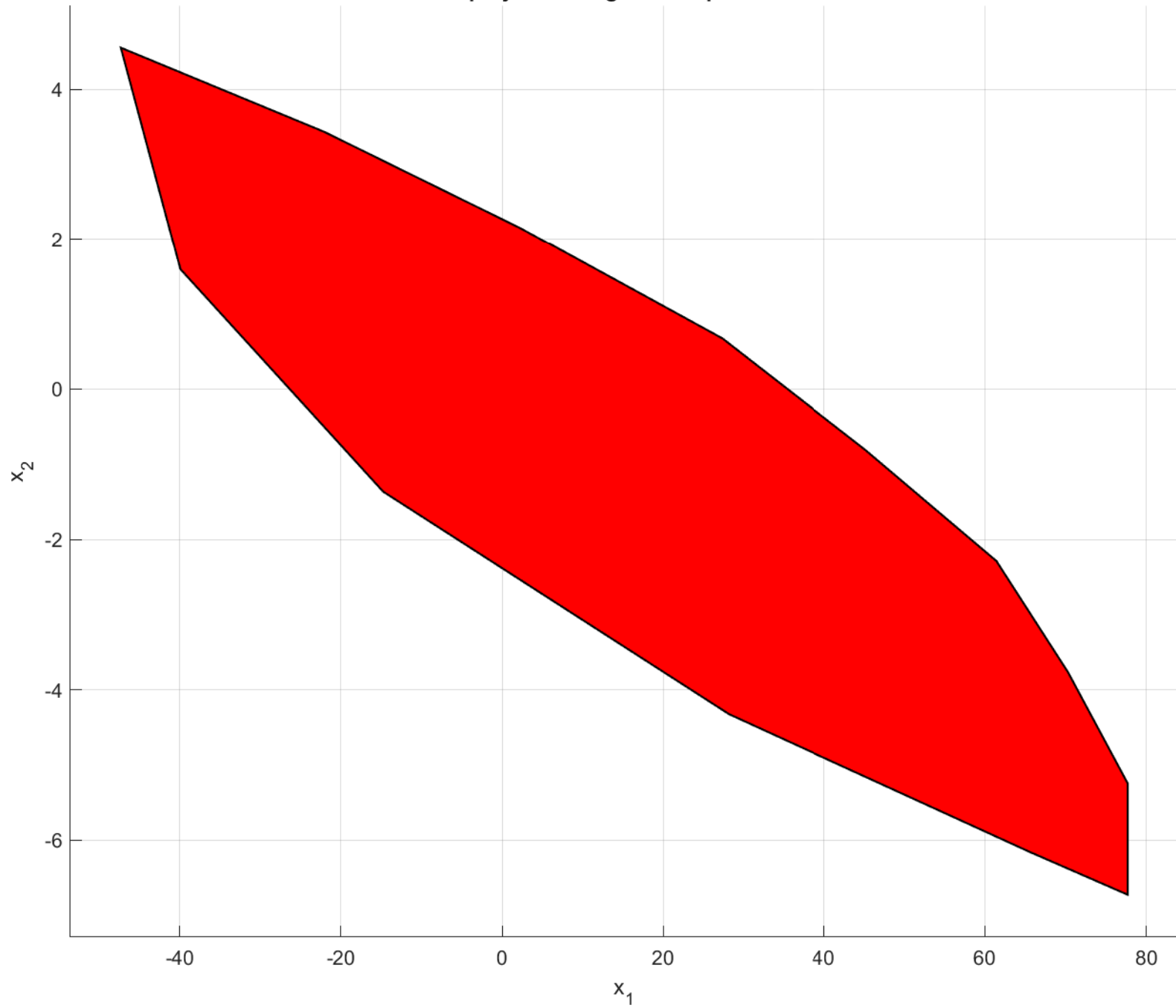
projecao integrador duplo N:3
