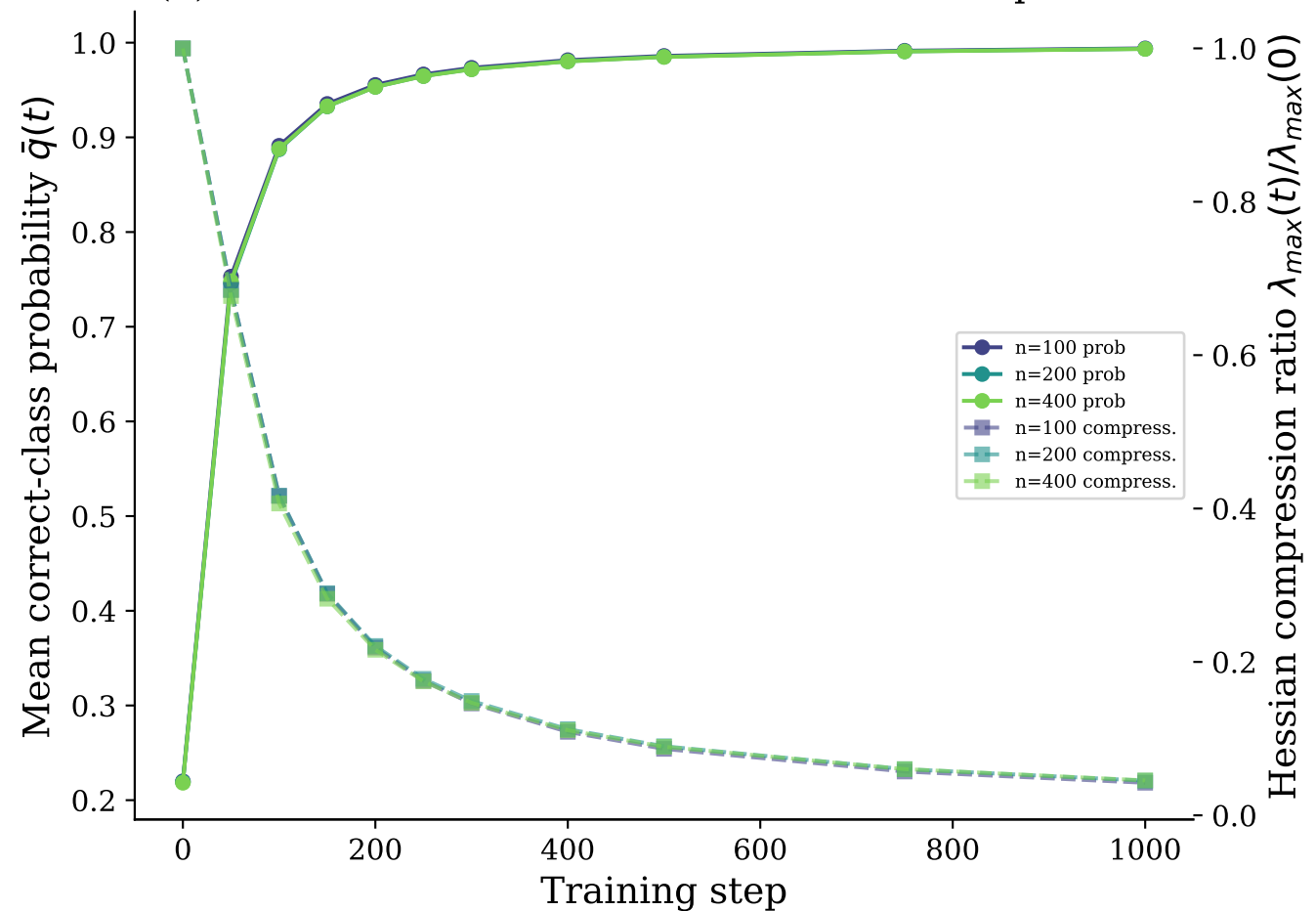
(d) Softmax concentration drives Hessian compression
