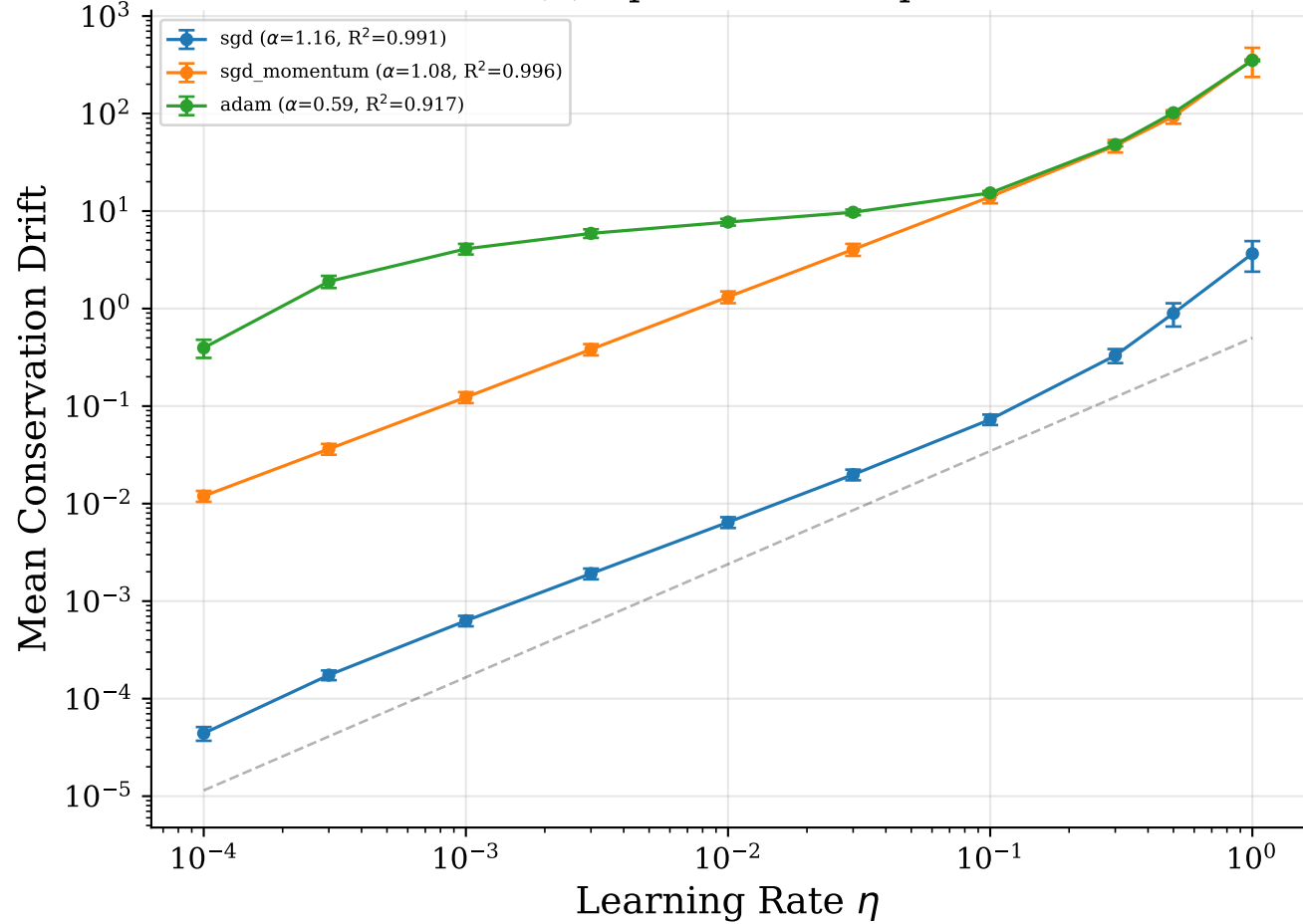
(d) Optimizer Sweep
