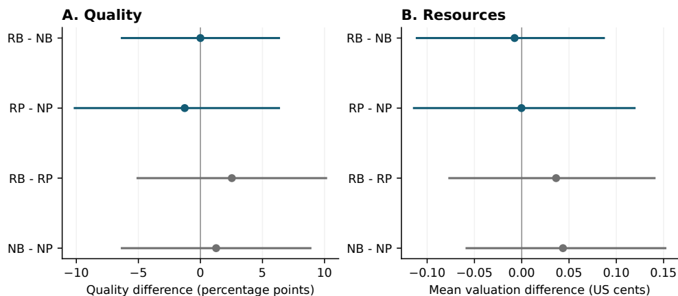
Рис. 5 Независимый эксперимент: парные разности качества (процентные пункты) и оценки по API-тарифам (центы США на кандидата), описательные 95% bootstrap-интервалы по задачам. Первые два контраста образуют основное семейство тестов качества; контрасты оформления описательные. RB/NB — ролевые/нейтральные заголовки, RP/NP — роли/этапы в сплошном тексте.
