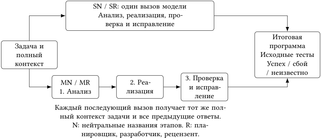
Рисунок 1. Схема сравнения одного и трех вызовов. Прямая базовая линия D использует один вызов без поэтапных инструкций. Оценивание выполняется после генерации, и тесты бенчмарка никогда не возвращаются в эти пять условий. Внутренние этапы одношагового режима являются инструкциями, а не отдельно наблюдаемыми выполнениями.
