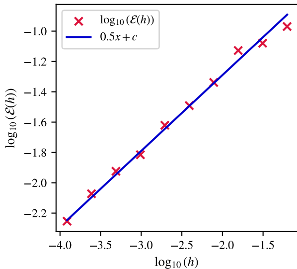
\mathcal{E}(h) for EES(2,7)
