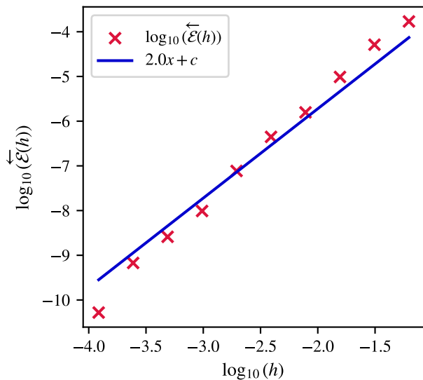
\overleftarrow{\mathcal{E}}(h) for EES(2,5)
