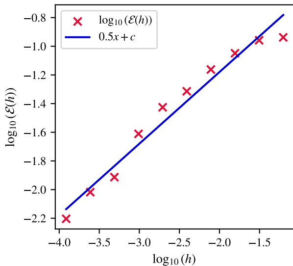
\mathcal{E}(h) for EES(2,5)
