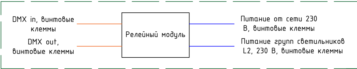
Подключение релейного DMX модуля, типовое
