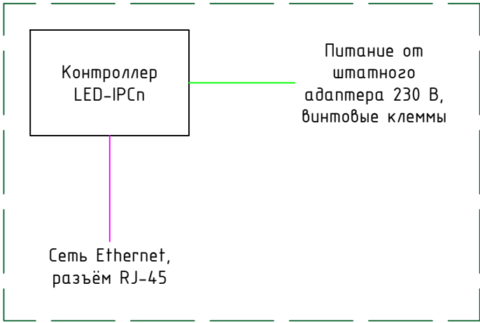
Подключение головного контроллера LED-IPСп
