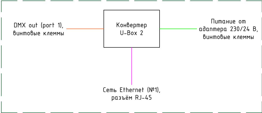
Подключение конвертера U-Box 2, типовое
