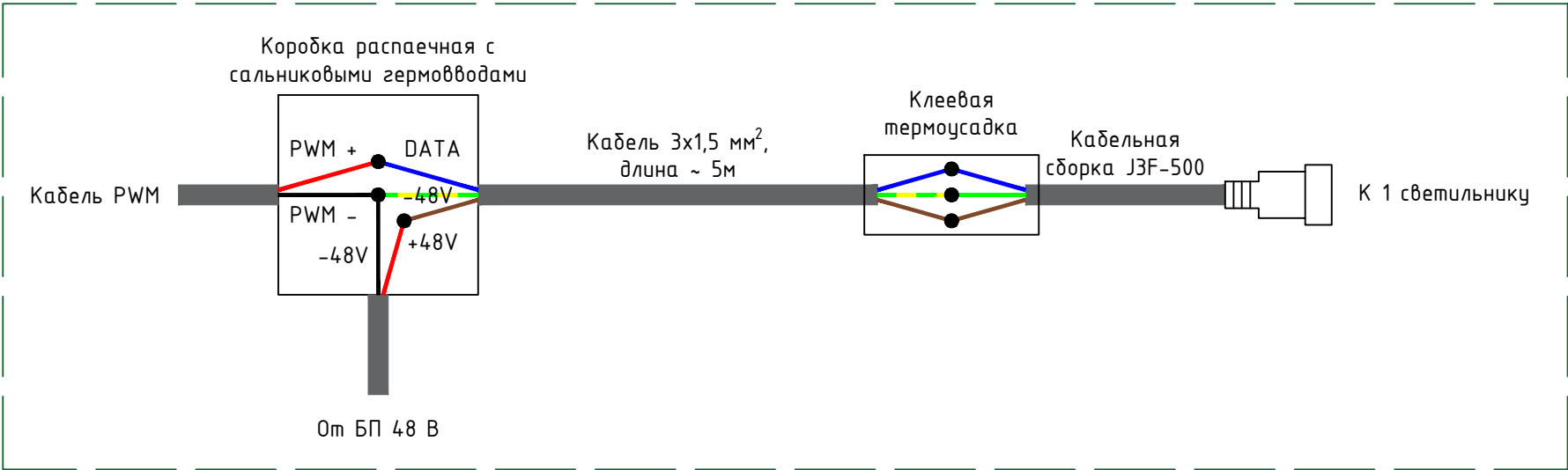
Подключение питания и управления к 1 светильнику (тип L1.X), типовое
