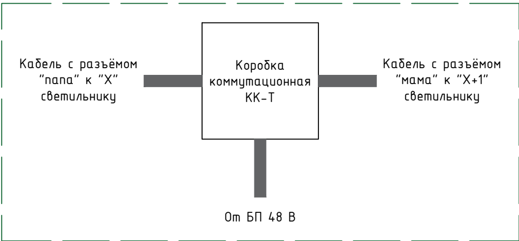
Подключение питания "в разрыв" линии светильников (тип L1.X), типовое
