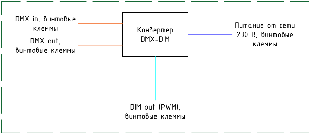
Подключение конвертера DMX-DIM, типовое
