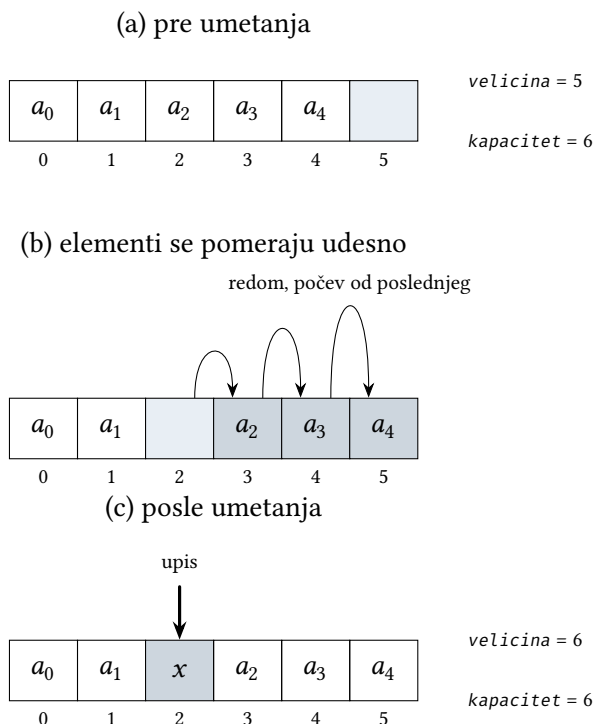
Slika 3.3: Umetanje elementa na poziciju 2. Elementi od pozicije umetanja do kraja niza pomeraju se za jedno mesto udesno, počev od poslednjeg, a zatim se novi element upisuje na oslobođeno mesto.
