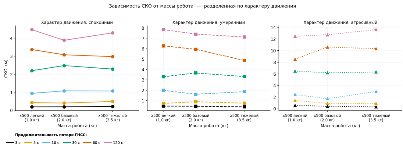
Рисунок 4.4 — Зависимость СКО от массы робота, разбивка по профилю полёта
