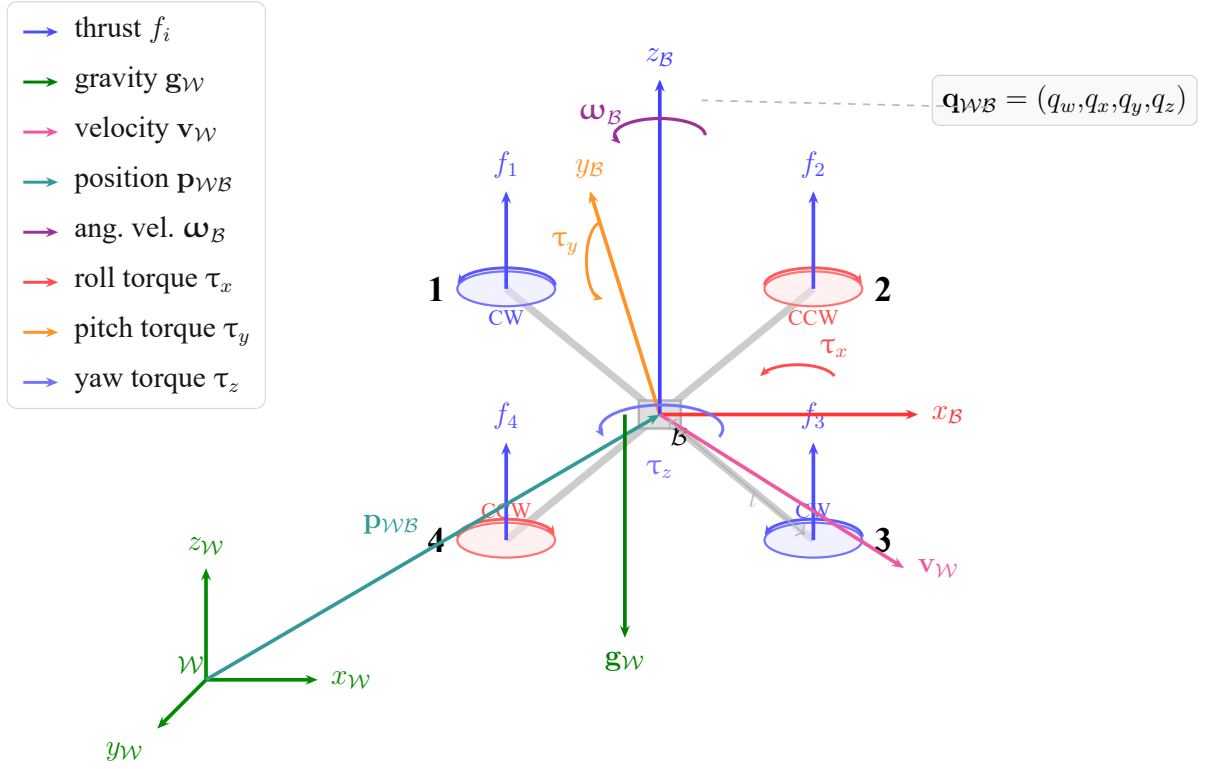
Рисунок 2.1 — Кинематика и динамика квадрокоптера. Инерциальная система координат \mathcal{W} (зелёная) и связанная система координат \mathcal{B} (красная/оранжевая/синяя) с положением центра масс \mathbf{p}_{WB} (бирюзовый), линейной скоростью \mathbf{v}_W (пурпурный), угловой скоростью \boldsymbol{\omega}_B (фиолетовый), силами тяги отдельных роторов f_i = k_T \omega_i^2 (синие стрелки), силой тяжести \mathbf{g} (зелёный), моментами крена, тангажа и рыскания \tau_{x,y,z} и кватернионом ориентации \mathbf{q}_{WB} . Роторы 1 и 3 вращаются по часовой стрелке (CW, синие эллипсы), роторы 2 и 4 — против часовой стрелки (CCW, красные эллипсы).
