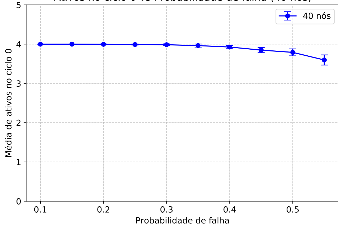
Ativos no ciclo 0 vs Probabilidade de falha (40 nós)
