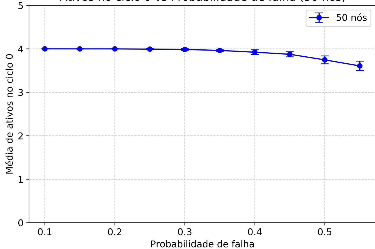
Ativos no ciclo 0 vs Probabilidade de falha (50 nós)
