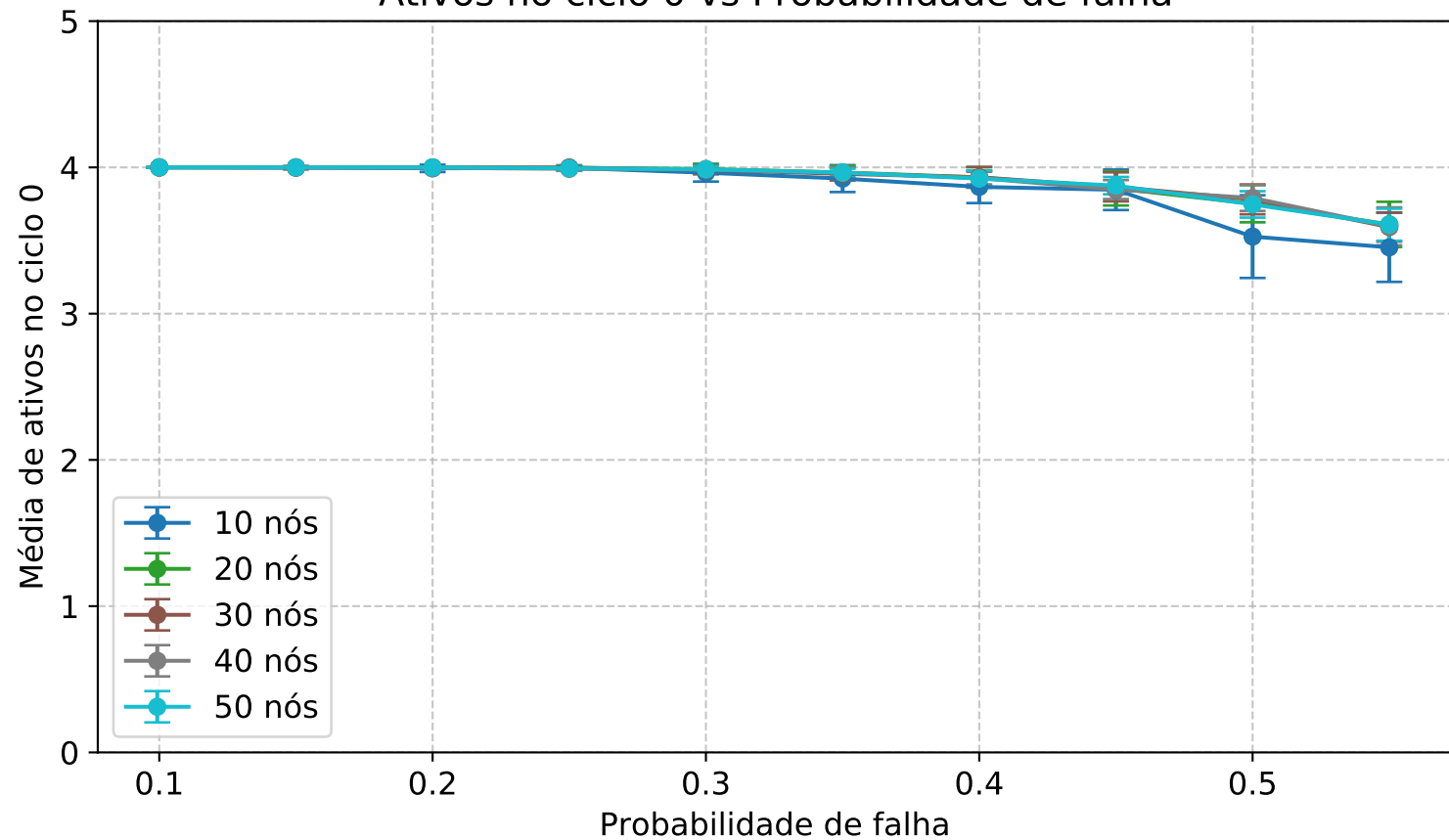
Ativos no ciclo 0 vs Probabilidade de falha
