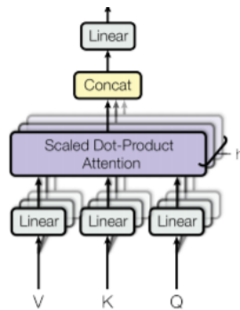
Слика 18: Multiheadattention
