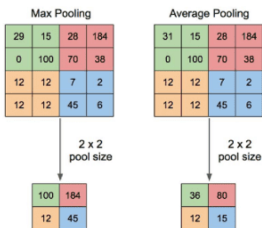
Слика 9: *Pooling* операција
