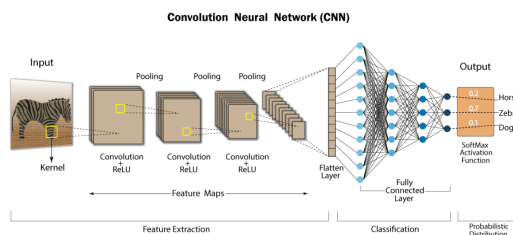
Слика 8: Архитектура конволуционе мреже
