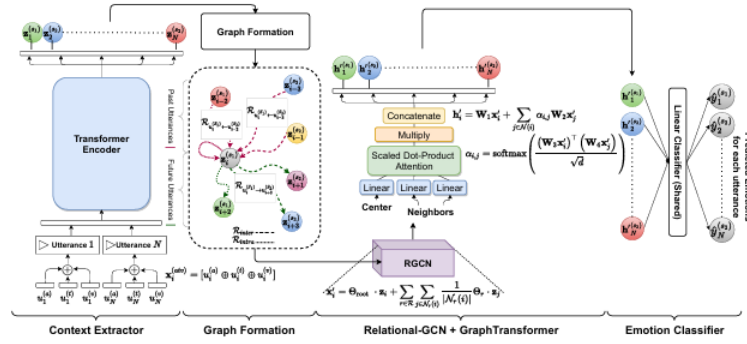
Слика 31: Архитектура COGMEN а
