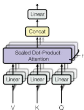
Слика 18: Multiheadattention
