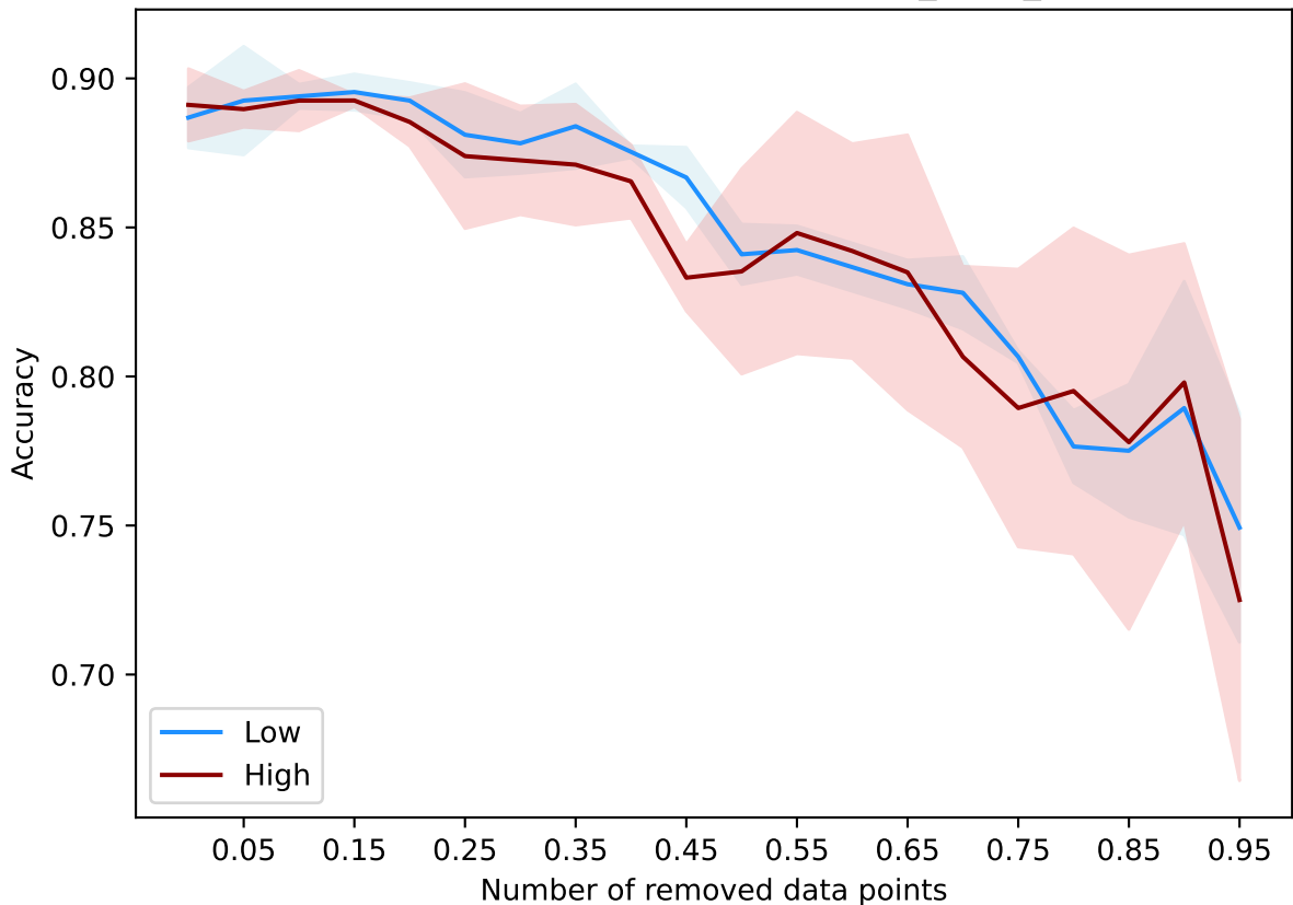
RandomEvaluator() - nomaoworst_class_acc
