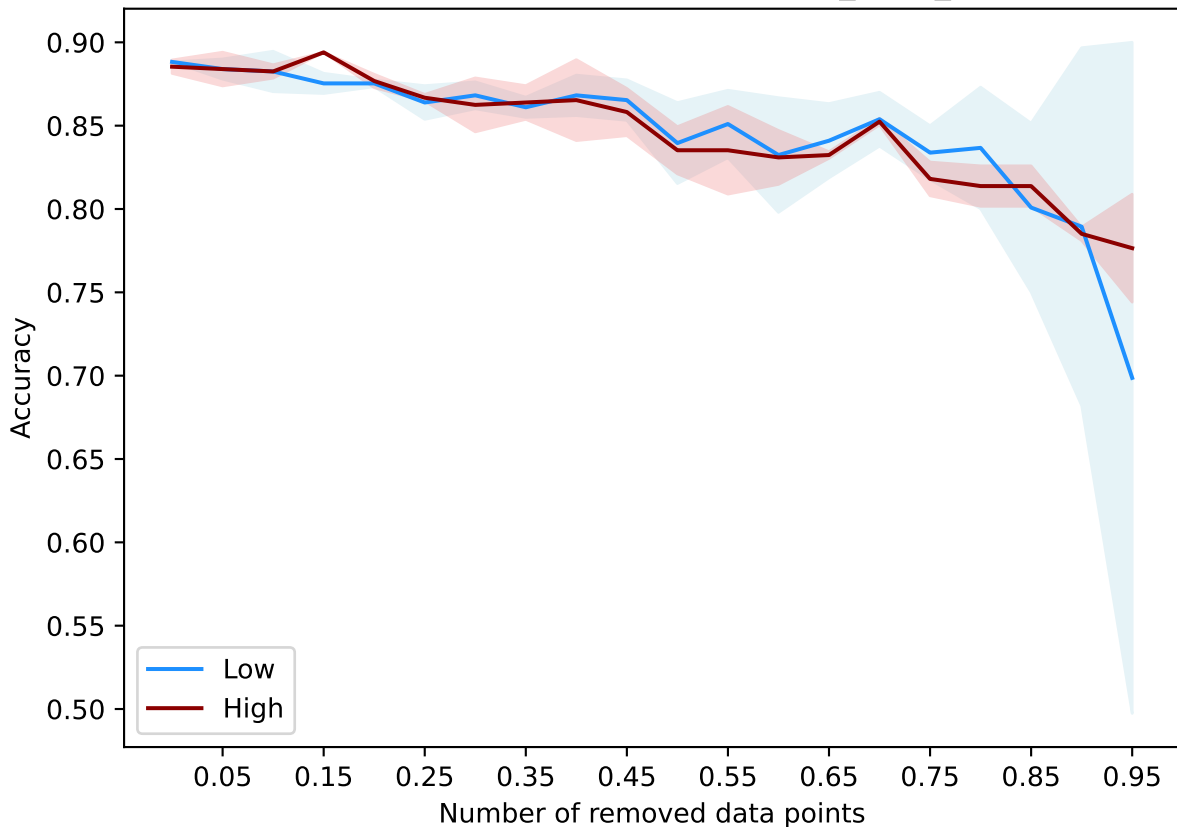
RandomEvaluator() - nomaoworst_class_acc
