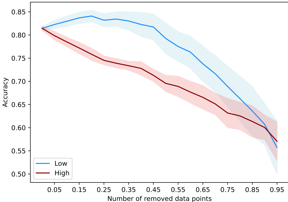
DataBanzhaf(num_models=1000) - pol
