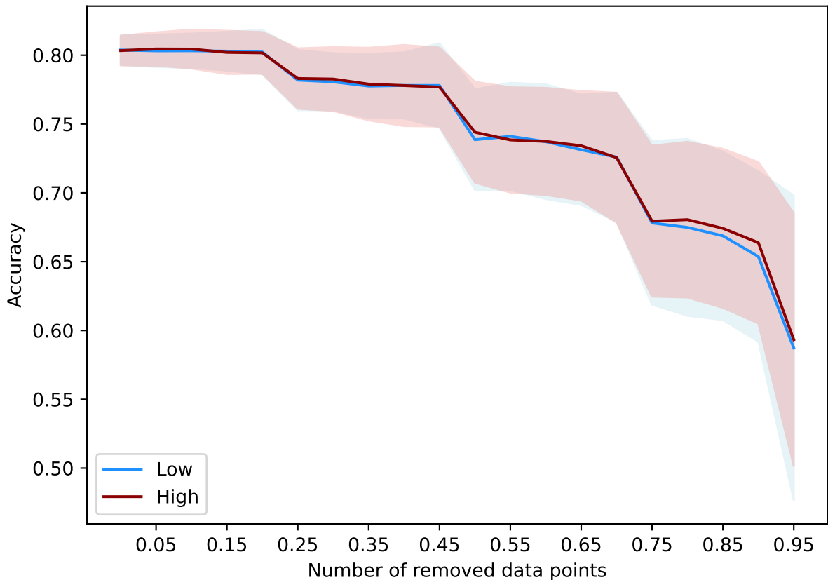
RandomEvaluator() - pol
