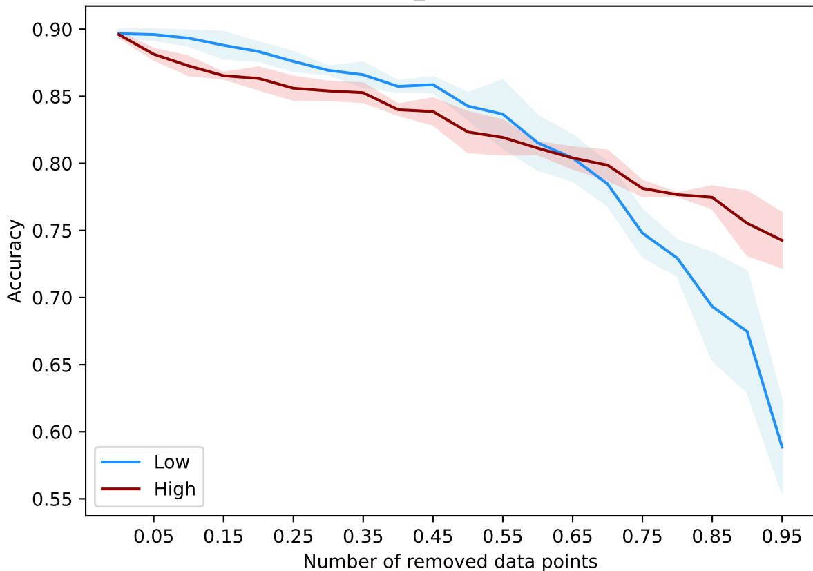
DataBanzhaf(num_models=1000) - nomao
