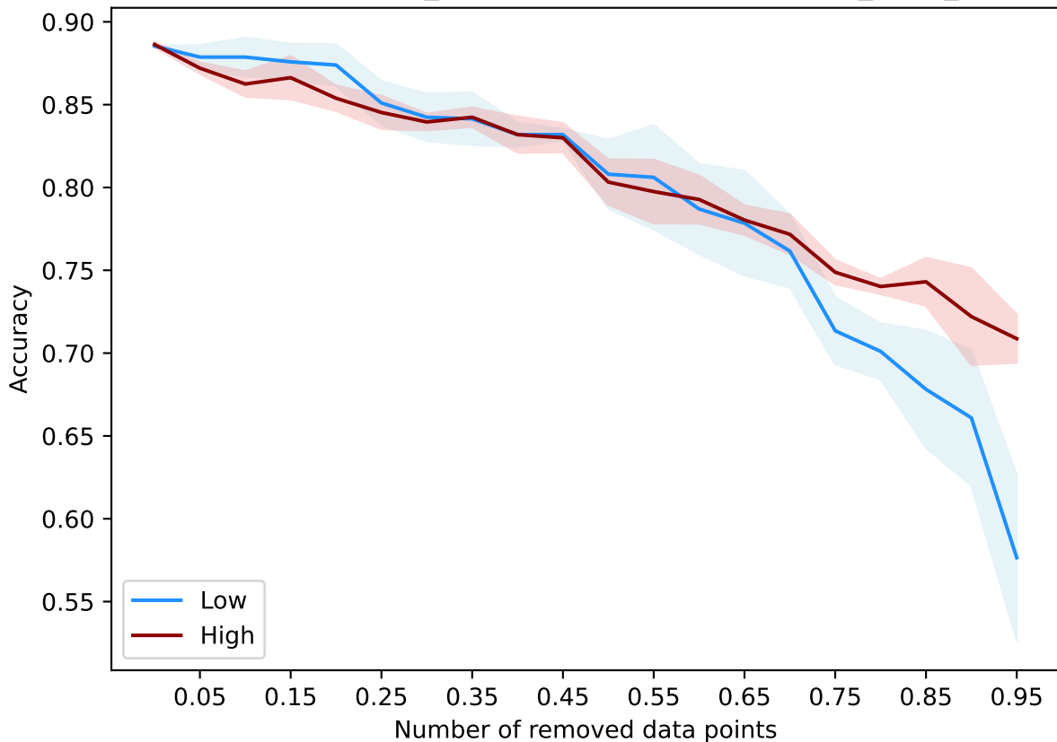
DataBanzhaf(num_models=1000) - nomaoworst_class_acc
