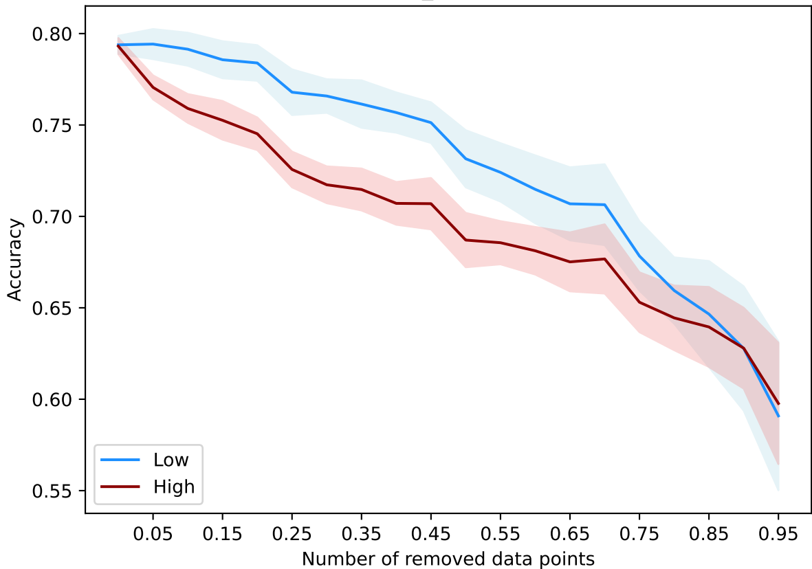
DataBanzhaf(num_models=1000) - adult
