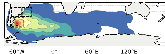
After: EOF 4 (n=203)
