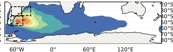
Before: EOF 2 (n=450)
