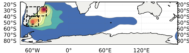
Before: EOF 1 (n=492)
