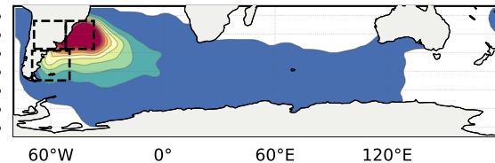
Before: EOF 4 (n=443)
