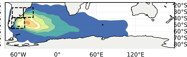
After: EOF 2 (n=260)
