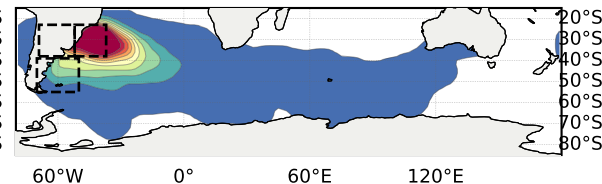
After: EOF 3 (n=281)
