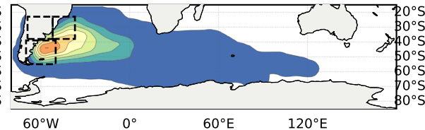
Before: EOF 3 (n=430)
