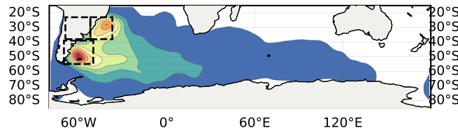
After: EOF 1 (n=286)
