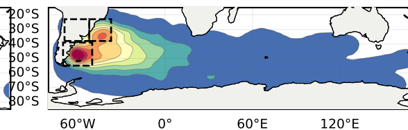
After: EOF 3 (n=290)
