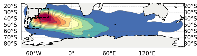
After: EOF 1 (n=311)
