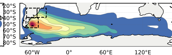
After: EOF 2 (n=306)
