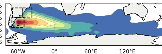
After: EOF 4 (n=296)
