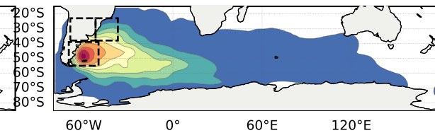
After: EOF 4 (n=329)
