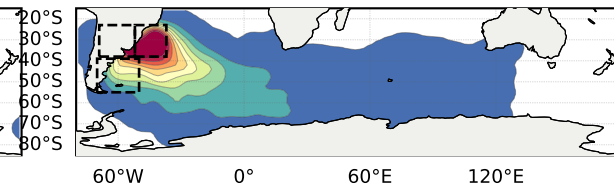
Before: EOF 4 (n=340)
