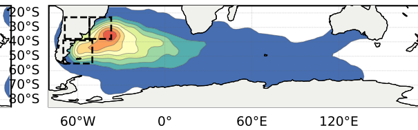
Before: EOF 2 (n=297)
