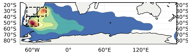
After: EOF 1 (n=323)
