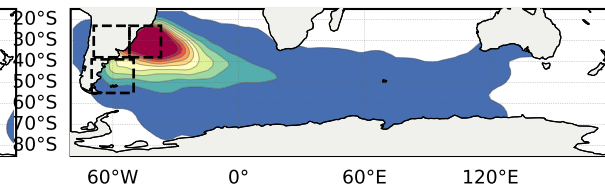
After: EOF 2 (n=338)
