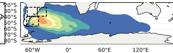
After: EOF 3 (n=330)
