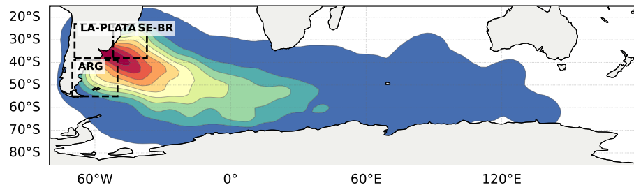
(D) EOF 4 (n=291)
