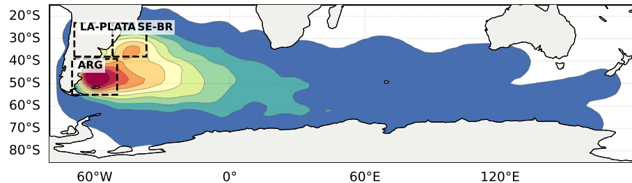
(B) EOF 2 (n=314)
