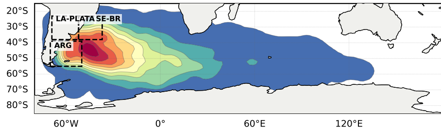
(B) EOF 2 (n=320)
