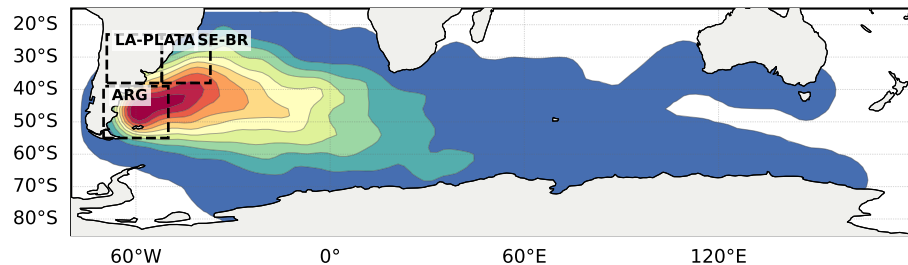
(D) EOF 4 (n=288)
