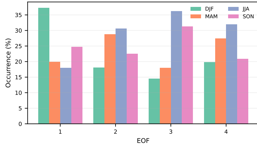
(D) Seasonal occurrences - EOF(-)
