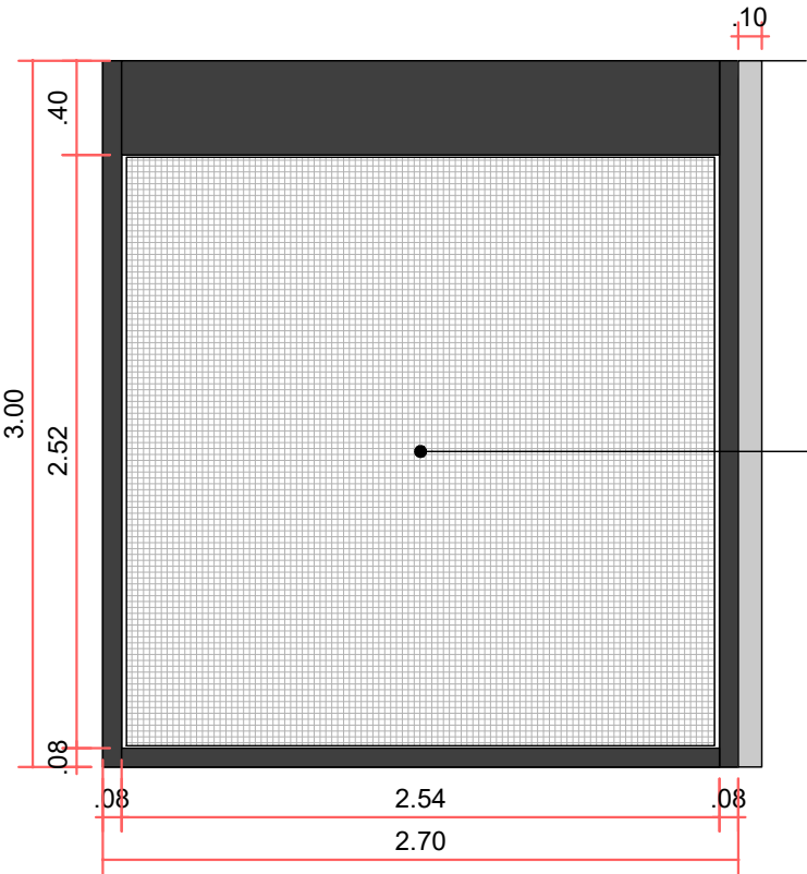
VISTA LATERAL DIREITA SEM ESCALA
