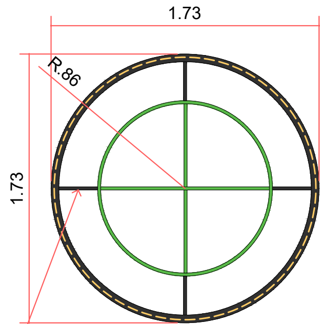
PLANTA PEÇA MONTADA
