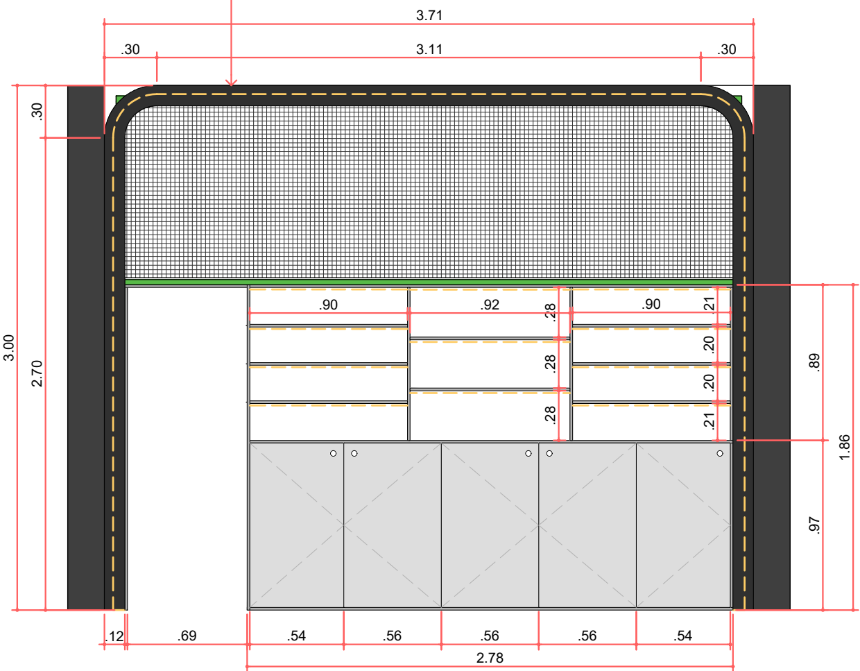
VISTA FRONTAL ACABADA
