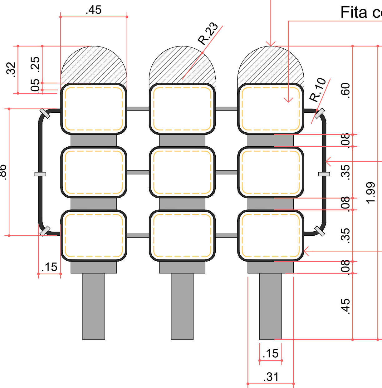
VISTA FRONTAL SEM ESCALA
