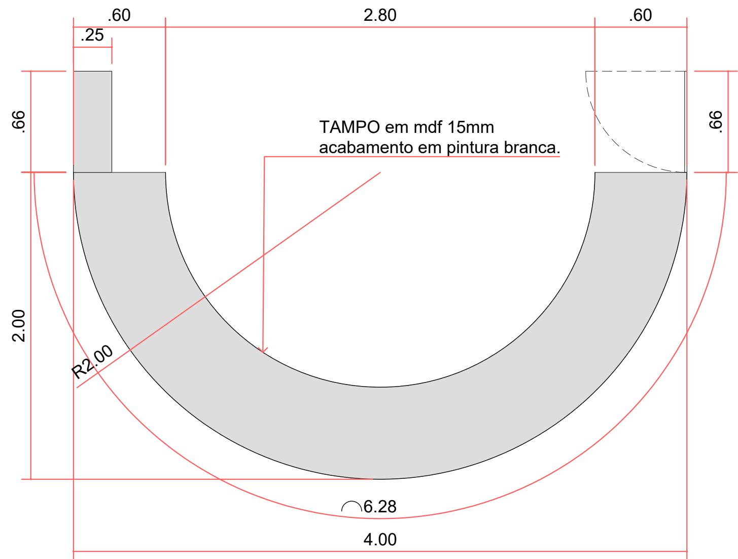
PLANTA TOPO
