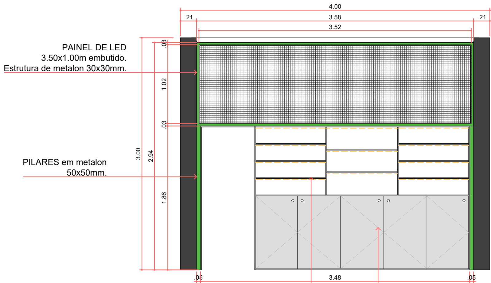
VISTA FRONTAL ESTRUTURA
