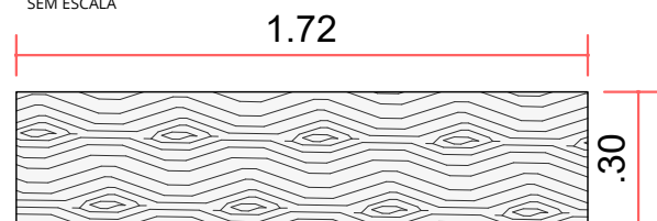
VISTA FRONTAL METALON
