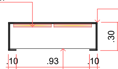
VISTA INTERNA FUNCIONAMENTO DA CAIXA
