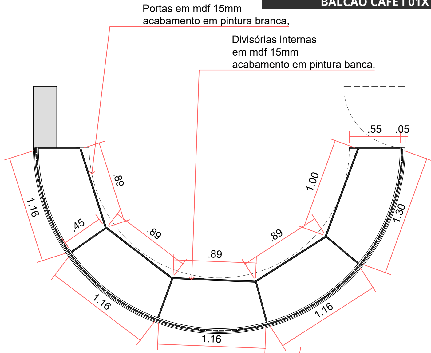
PLANTA BAIXA
