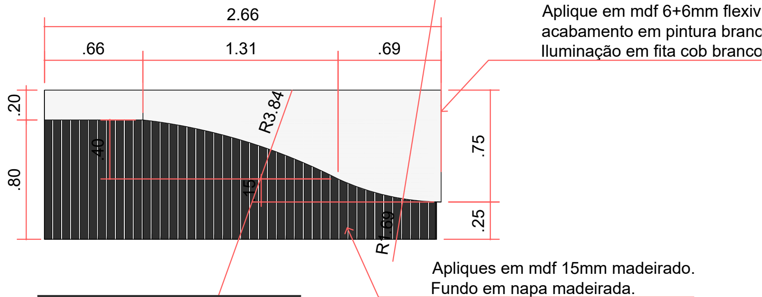
VISTA LAT. ESQUERDA
