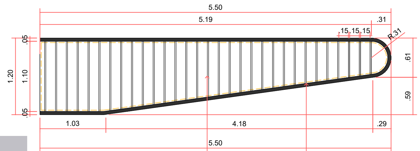
VISTA LATERAL
