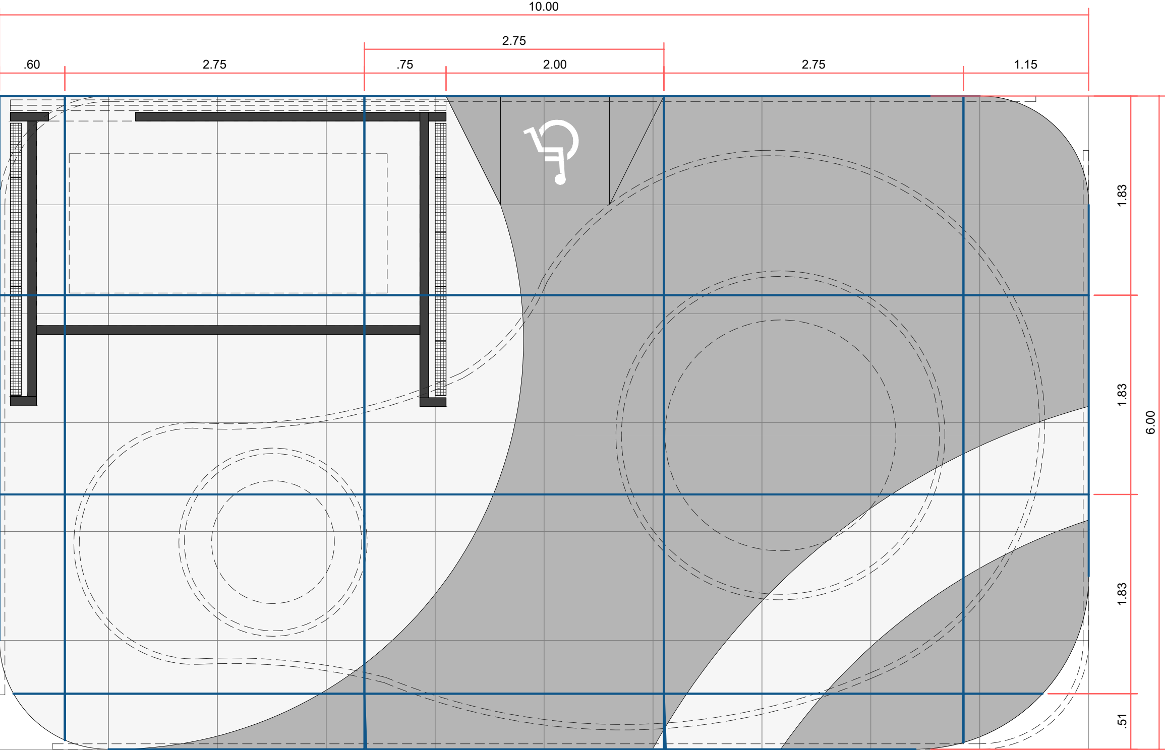
PLANTA PISO MAPA DE CHAPAS SEM ESCALA
