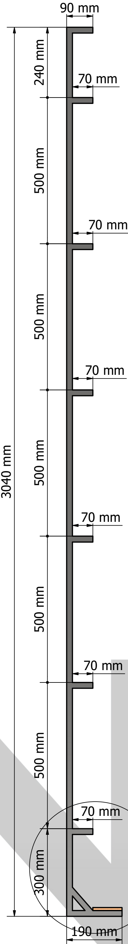
VISTA LATERAL
