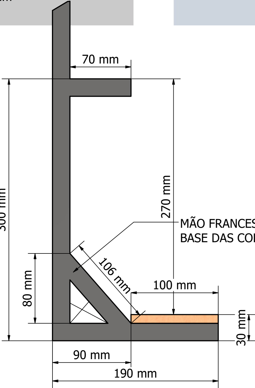
DET. 1
