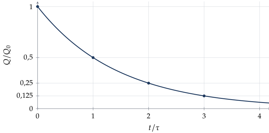
Figura 16. Problema 5. Decaimiento radiactivo: cada periodo de vida media la cantidad se reduce a la mitad.
