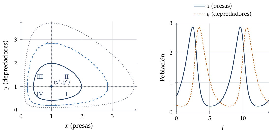
(a). Órbitas H = c ( c = 2,3; 2,8; 3,4 ), con el sentido de recorrido y las cuatro fases.
